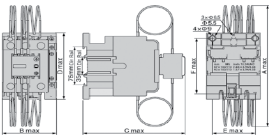
GDC-25,32,43
