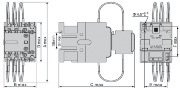
GDC-63, 95, 115
