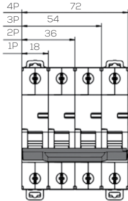
Boyutlar (mm)
