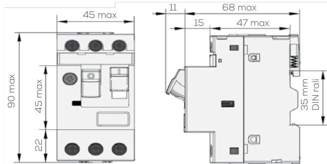
Boyutlar (mm)
