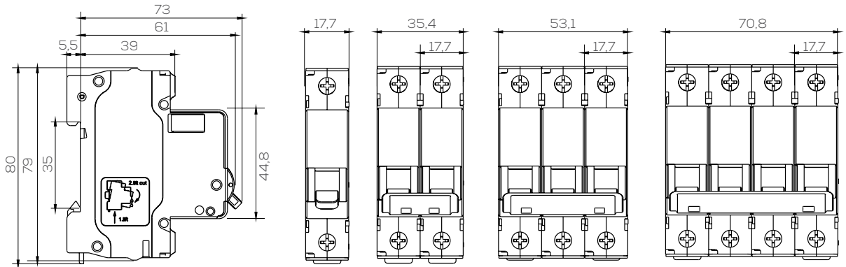
Boyutlar (mm)
